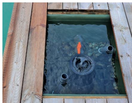
Der schwimmende Skimmer saugt das Oberflächenwasser an und filtert größere Schmutzpartikel heraus. Da er schwimmt, ist er relativ einfach zu entnehmen und zu reinigen.
